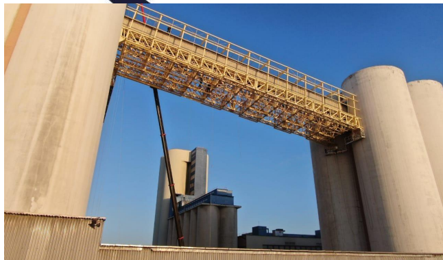
PASSARELA MUCURIBE - M DIAS BRANCO - M.DIAS 40m de comprimento / 40m de nível do solo Fortaleza - CE
